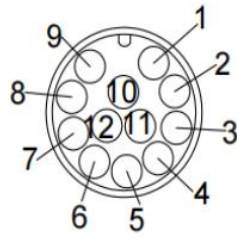
M12公头P1端正视图
